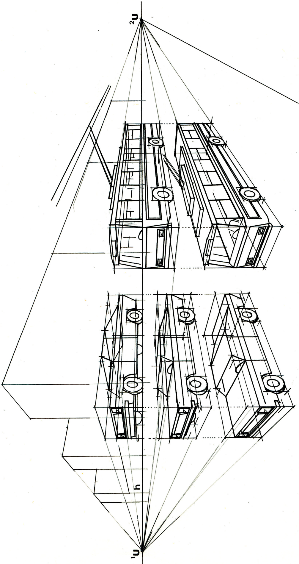
Obr. 252. Konstrukce tvaru dopravního prostředku vzhledem k poloze horizontu
